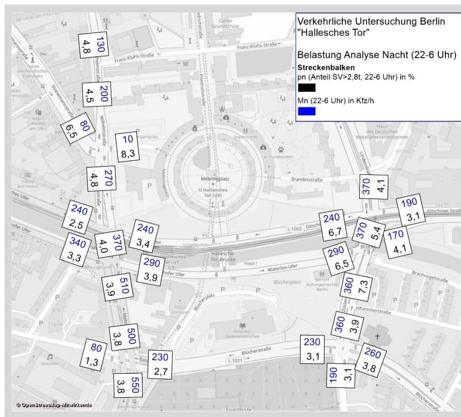
Analyse: maßgebende Verkehrsstärke und Lkw-Anteil in der Nacht
