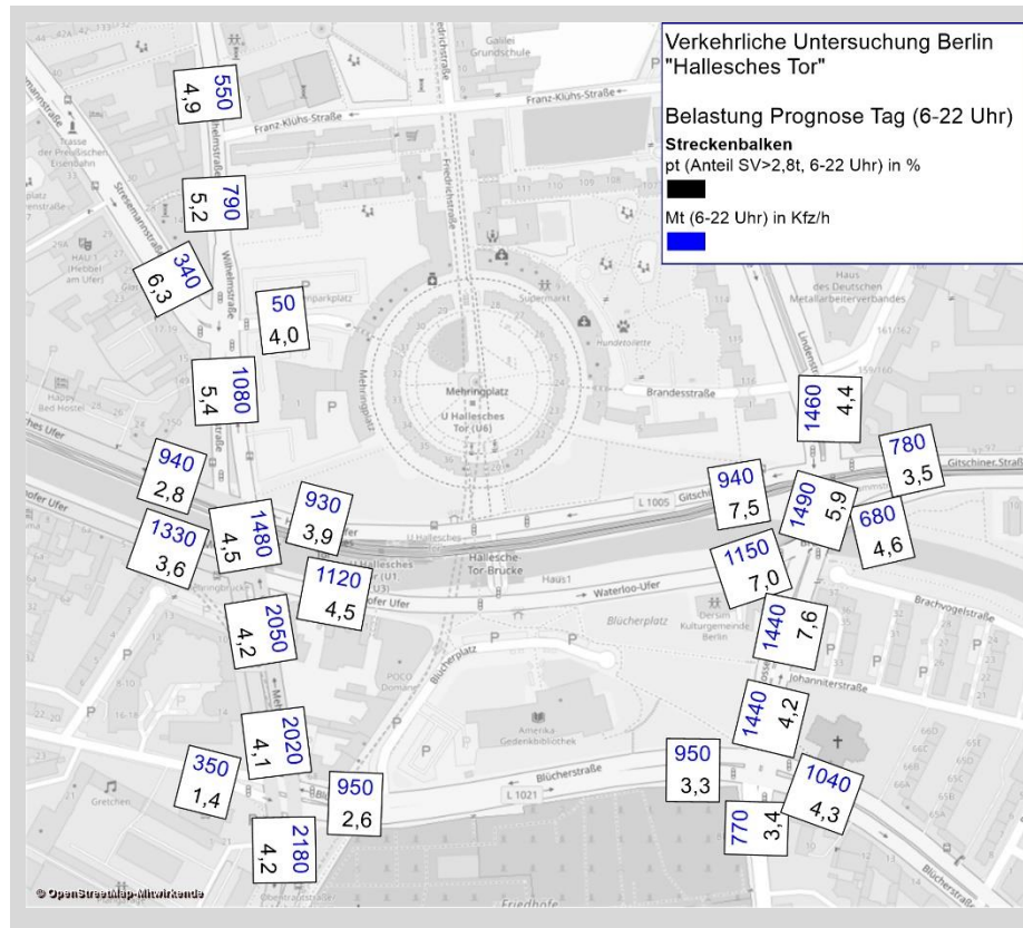
Prognose: maßgebende Verkehrsstärke und Lkw-Anteil am Tag
