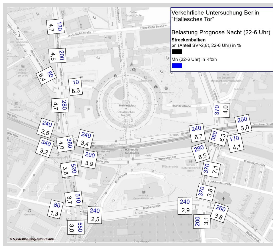
Prognose: maßgebende Verkehrsstärke und Lkw-Anteil in der Nacht
